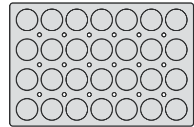
74102-02 SEMI SPHERE 28 cav. 36 · Ø 72 mm. / 1,42" · Ø 2,83"
