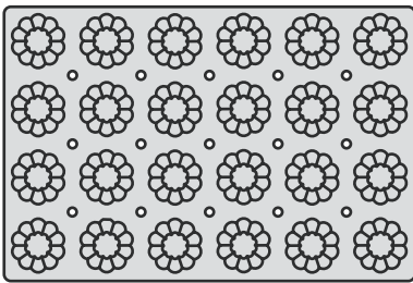
74102-08 BRIOCHETTE 24 cav. 36 · Ø 78 mm. / 1,42" · Ø 3,07"
