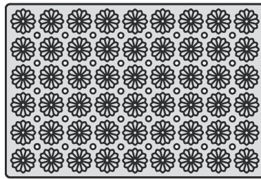
74102-04 CANNELE BORDELAIS 54 cav. 49 · Ø 58 mm. / 1,93" · Ø 2,28"
